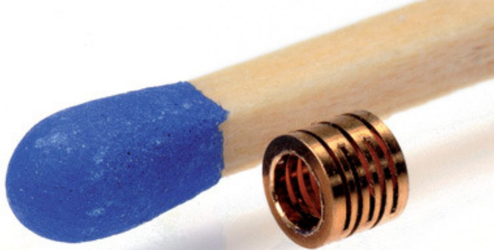
Das Streichholz unterstreicht die Winzigkeit des Drehlagers für das Headshell. Es handelt sich um ein vorgespanntes Doppelschräg-Kugellager
